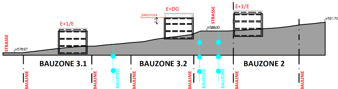
SYMBOLSCHNITT/ GELÄNDE DURCH ABSCHNITT-A DER BAUZONEN 3.1; 3.2 UND 2
